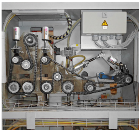
Les chaînes d'une installation de tronçonnage, avec avancement à rouleaux, sont lubrifiées en permanence et en même temps nettoyées grâce à trois graisseurs simalube incorporant des brosses.
