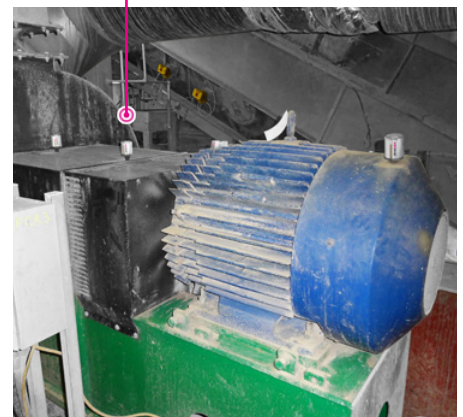
Der FGR Ventilator wird von simalube 60ml geschmiert.
